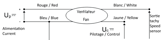
Schéma de branchement / Connection diagram / Anschlussplan N° II
