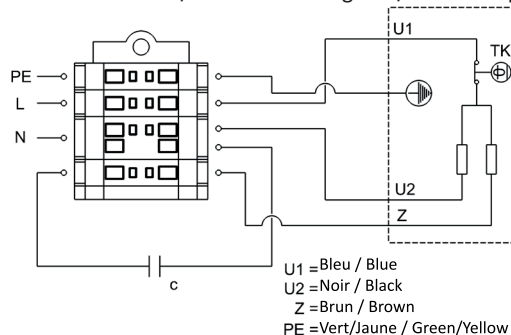
Schéma de branchement / Connection diagram / Anschlussplan N° IV
