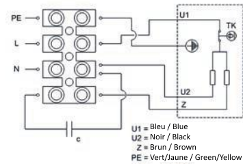
Schéma de branchement / Connection diagram / Anschlussplan N° III
