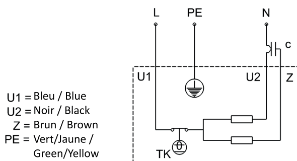
Schéma de branchement / Connection diagram / Anschlussplan N° II
